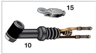
Corpo da tocha para SR 18 com gatilho
